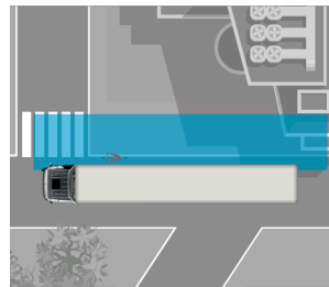
Actros con assistente alla svolta S1R (2 sensori a corto raggio rilevano un'area di 3,75 m di larghezza e 18,75 m di lunghezza)
